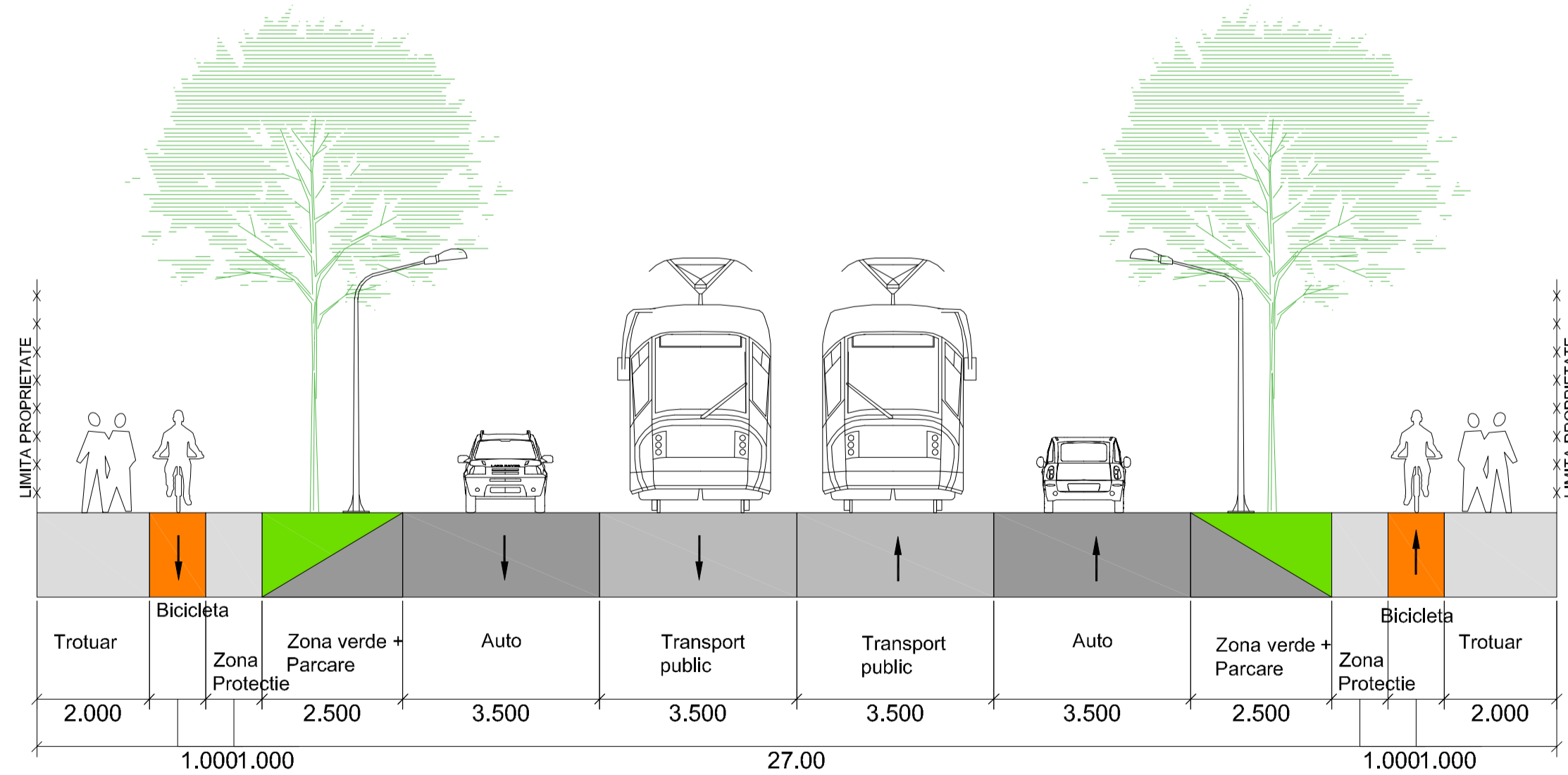
Profil Transversal 4 -lățime 26m
